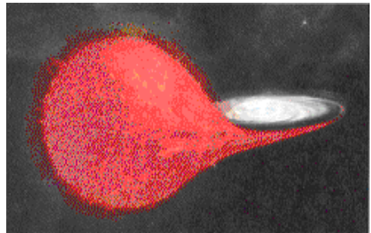
Uma supernova (estrela no fim de ciclo)
