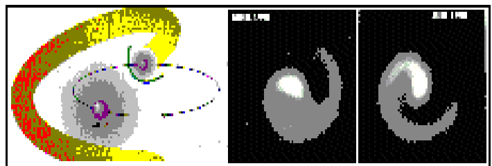
Uma estrela dupla e o movimento do desdobramento
